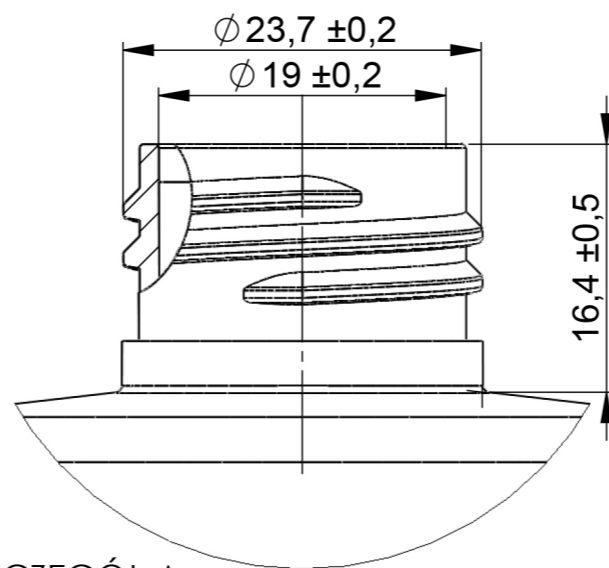
SZCZEGÓŁ A SKALA 2 : 1
