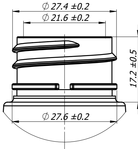
SZCZEGÓŁ A SKALA 2 : 1
