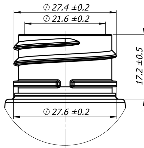
SZCZEGÓŁ A SKALA 2 : 1
